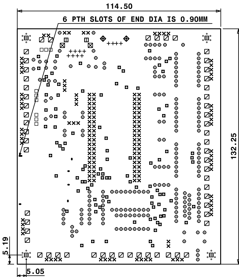
Drill Report : Layer E453774-60
